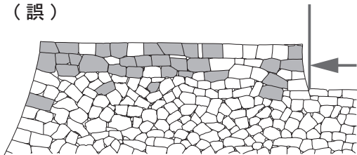
図版54 天守台石垣立面図 赤字が加筆・修正箇所
