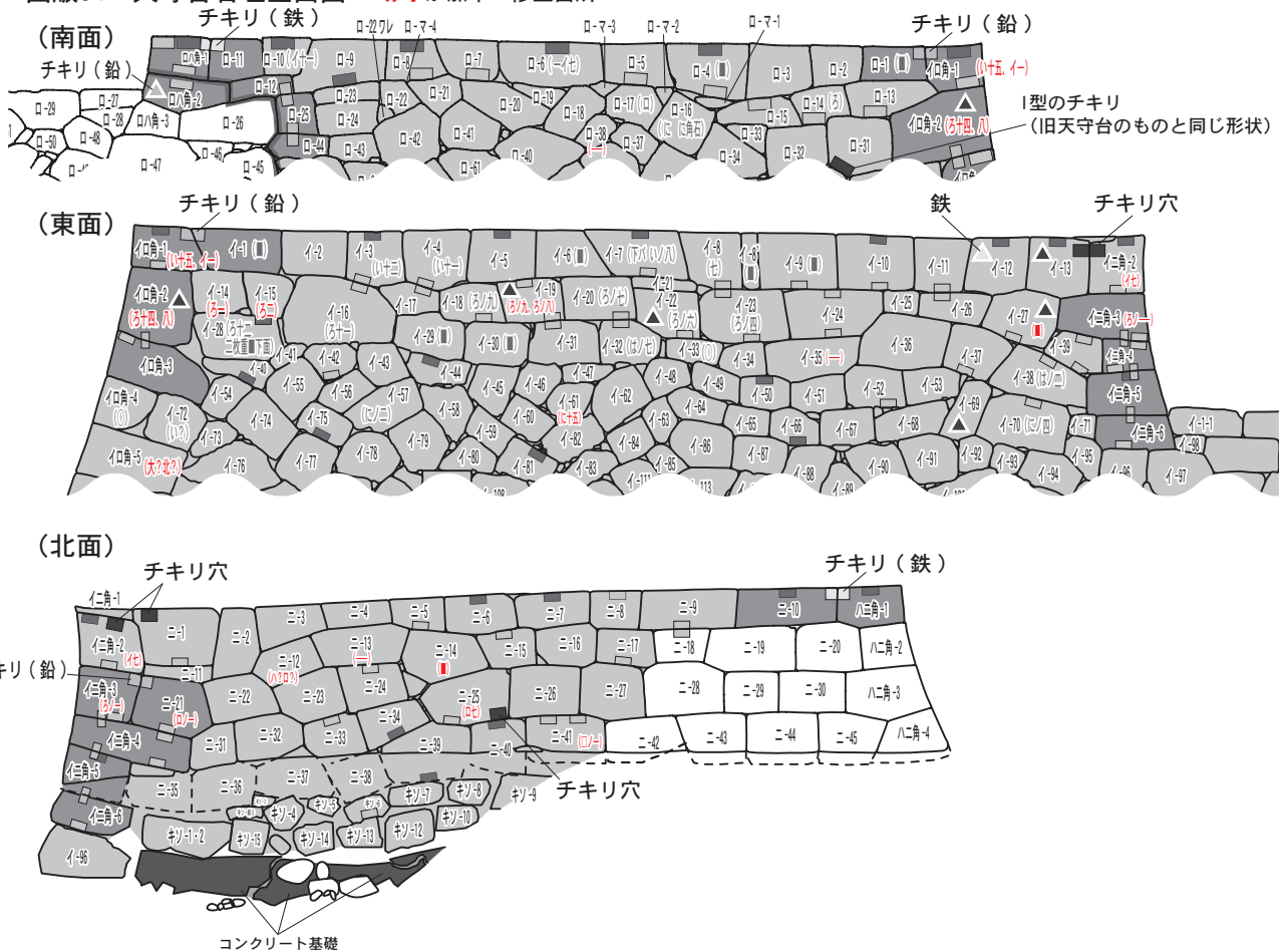
図版54 天守台石垣立面図 赤字が加筆・修正箇所
