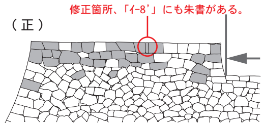
図版52 弘前城跡本丸東側石垣 朱書のある築石の分布状況（天端石～4石目まで）
