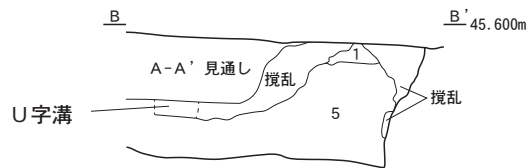
P105 図版 70 本丸放水銃付け替え掘削範囲図 よりセクション B
