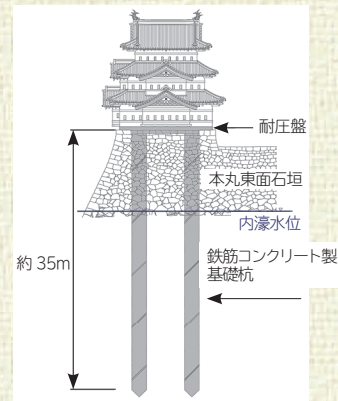
▲天守基礎耐震補強イメージ図(※3)
