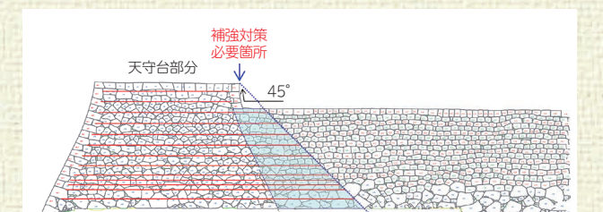
▲ジオテキスタイル工法範囲(赤線)(※4)
